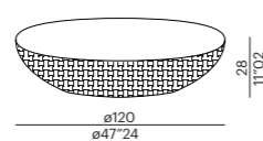
tavolo basso - low table TB-5 KUOIO
