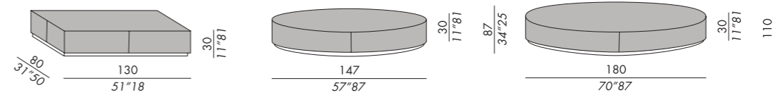
tavolo basso - low table TB-40 METAL tavolo basso - low table TB-50 METAL tavolo basso - low table TB-60 METAL tavolo basso - low table TB-35R METAL
