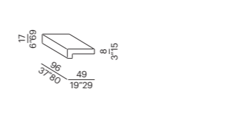
piano tavolo basso terminale - top for end-unit low table 49
