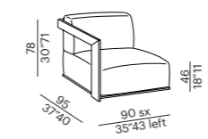
terminale - end unit
