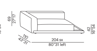
terminale angolo con tavolo basso - corner end unit with low table 205
