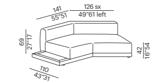
elemento asimmetrico con tavolo basso - asymmetrical unit with low table
