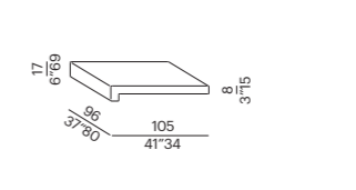
piano tavolo basso terminale - top for end-unit low table 105
