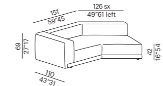
terminale asimmetrico - asymmetrical end unit
