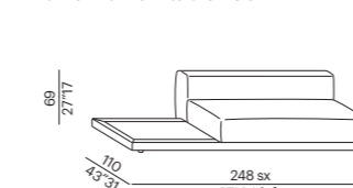
elemento con tavolo basso - unit with low table 250
